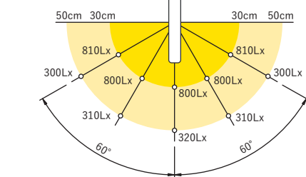
照度分布図
