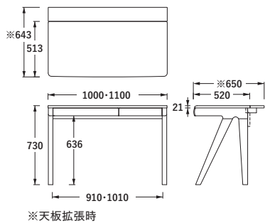
※天板拡張時
