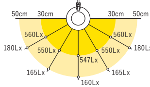
照度分布図
