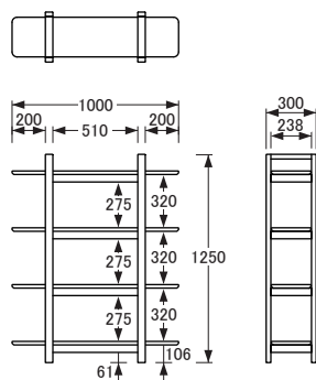
No.3800オープンラック〔W100〕
