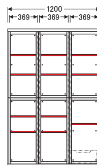
No.4600ボード ガラス戸〔W120〕
