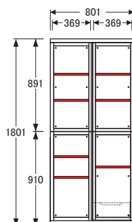
No.4600ボード ガラス戸〔W80〕
