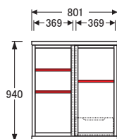
No.4600サイドボード 板戸〔W80〕
