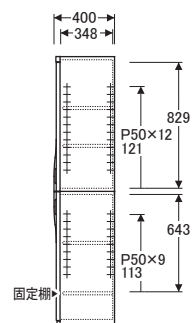
側面
