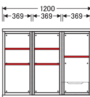
No.4600サイドボード ガラス戸〔W120〕
