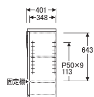
側面
