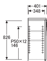
側面
