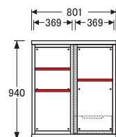
No.4600サイドボード ガラス戸〔W80〕
