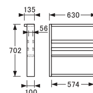
No.2000脚〔D65〕
