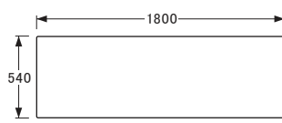
No.2000天板 〔180×54〕
