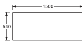
No.2000天板 〔150×54〕
