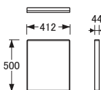
No.6000移動袖天板 [D50]
