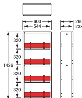
No.6000書棚 〔W60〕
