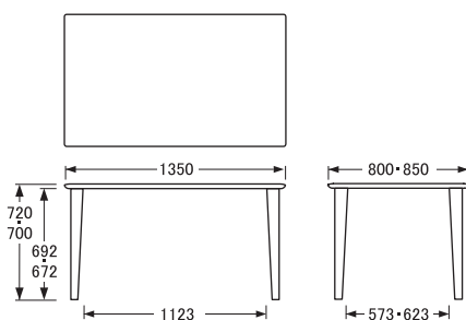
〔135×80×85×H70・72〕 側面
