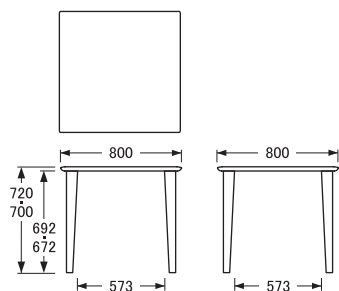
〔80×80×H70・72〕 側面
