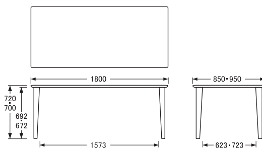
〔180×85×95×H70・72〕 側面
