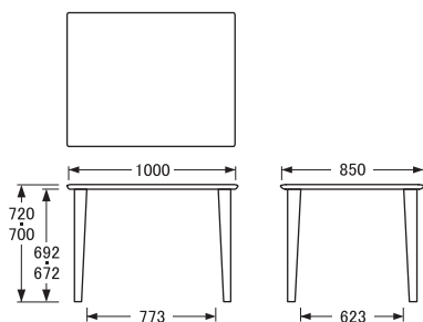
〔100×85×H70・72〕 側面
