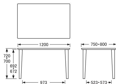
〔120×75×80×H70・72〕 側面
