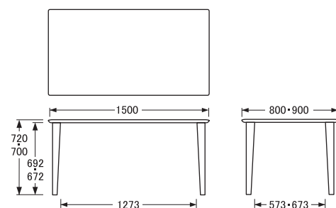
〔150×80×90×H70・72〕 側面
