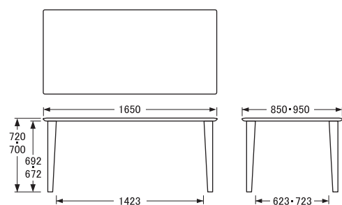
〔165×85×95×H70・72〕 側面
