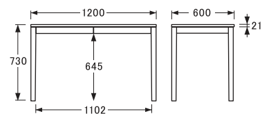
〔W120D60〕 側面
