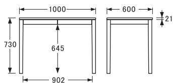
〔W100D60〕 側面
