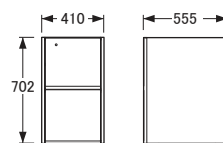
No.6000固定袖B〔D60〕
