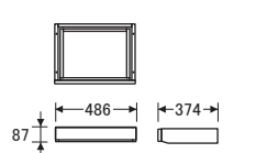
No.6000引出〔W49〕 〔引出内寸〕 W388×D306×H56
