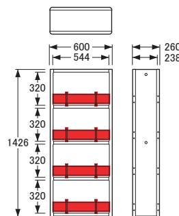
No.6000書棚 〔W60〕
