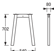
No.6000木製脚 〔D60〕
