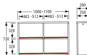
No.6000オープンラック 〔W100・W110〕
