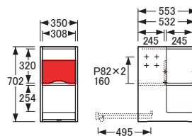
No.6000ラック脚〔D60〕
