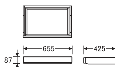
No.6000引出 〔W66〕 【引出内寸】 W551×D345×H56
