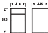
No.6000移動袖A 〔D50〕
