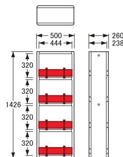
No.6000書棚 〔W50〕
