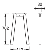
No.6000木製脚 〔D50〕
