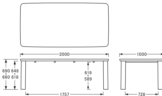
〔W200D100H66・69〕
