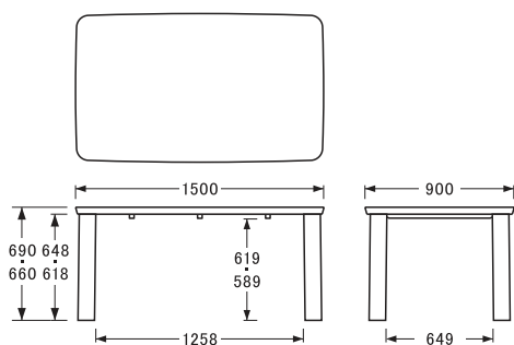
〔W150D90H66・69〕
