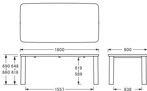
〔W180D90H66・69〕
