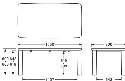
〔W165D90H66・69〕
