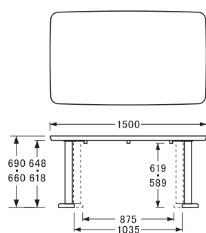
〔W150D90H66・69〕
