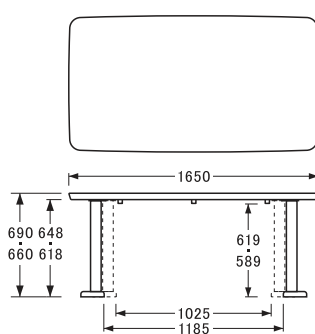
〔W165D90H66・69〕
