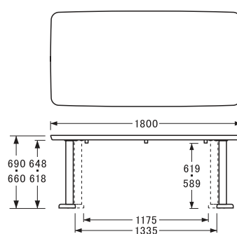
〔W180D90H66・69〕
