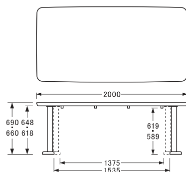
〔W200D100H66・69〕
