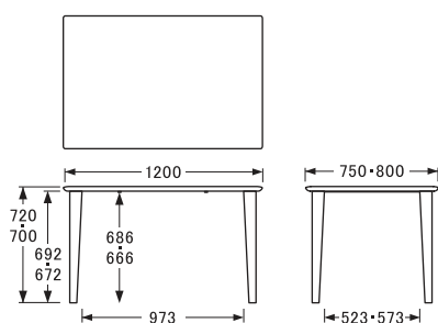
〔W120D75・80H70・72〕 側面
