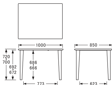
〔W100D85H70・72〕 側面
