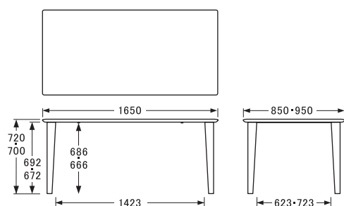
〔W165D85・95H70・72〕 側面
