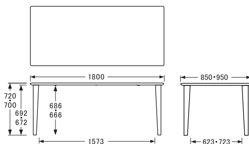
〔W180D85・95H70・72〕 側面
