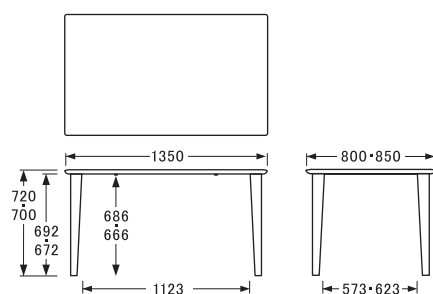
〔W135D80・85H70・72〕 側面
