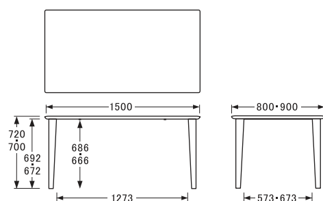
〔W150D80・90H70・72〕 側面
